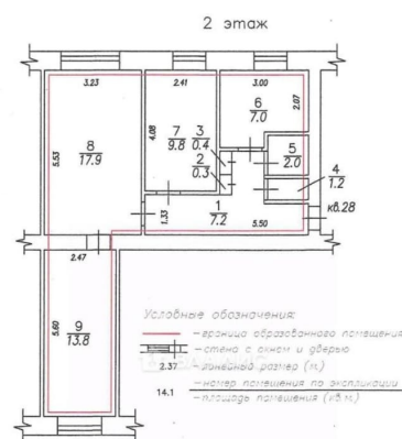
Экспликация к поэтажному плану
