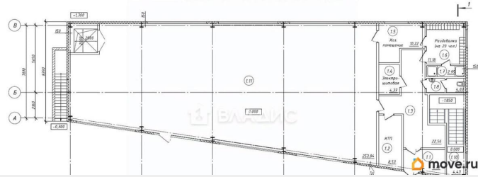
Отделочный план 1 этажа на отм. 0.000
